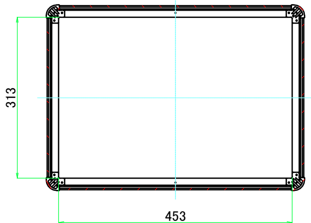
C-C ( 1 : 7.5 )
