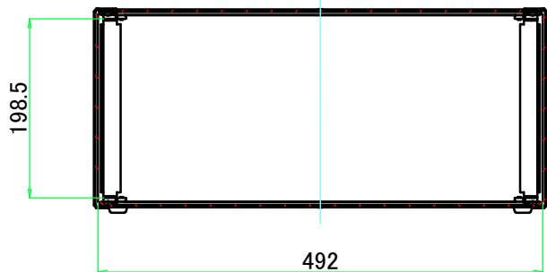
B-B ( 1 : 7.5 )
